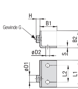
STAUFF GröÙe 1
